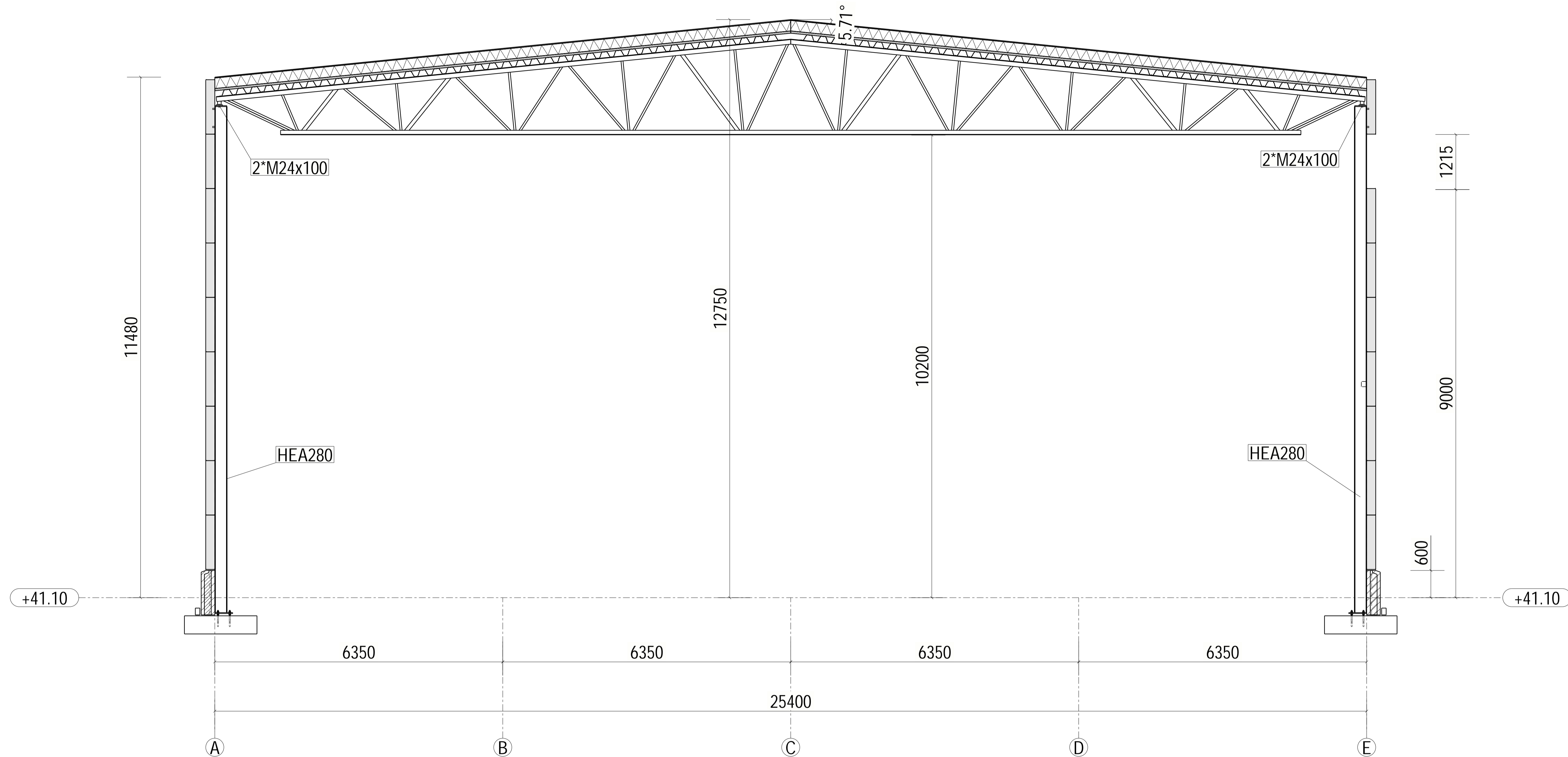
SEKTION 2-12 1:50
